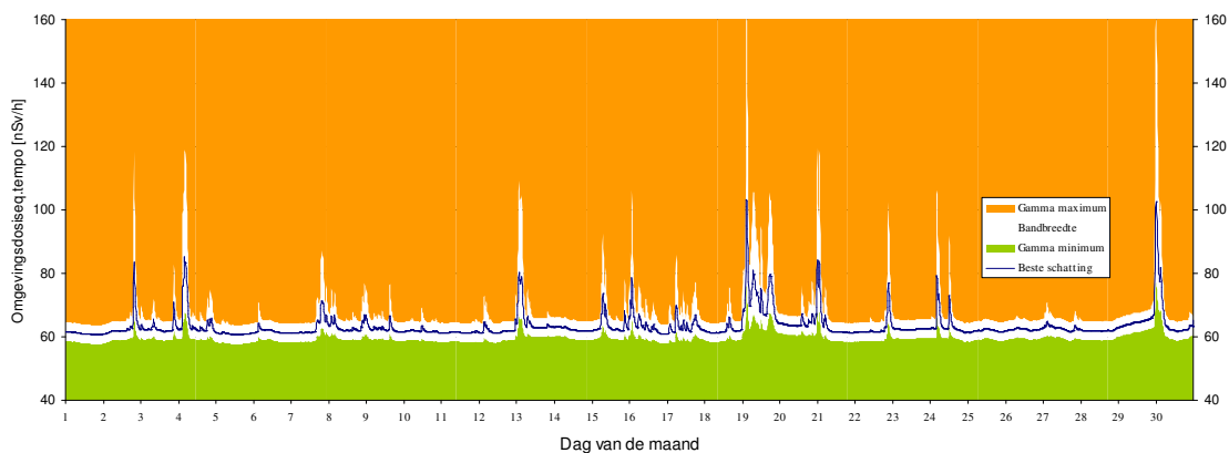
Figuur 9 Berekende tien-minuutwaarden van het omgevingsdosissequivalenttempo, gebaseerd op invoergegevens volgens Figuur 8. De achtergrondwaarde is gelijk gekozen aan die van NMR-lokatie Petten (1006).
