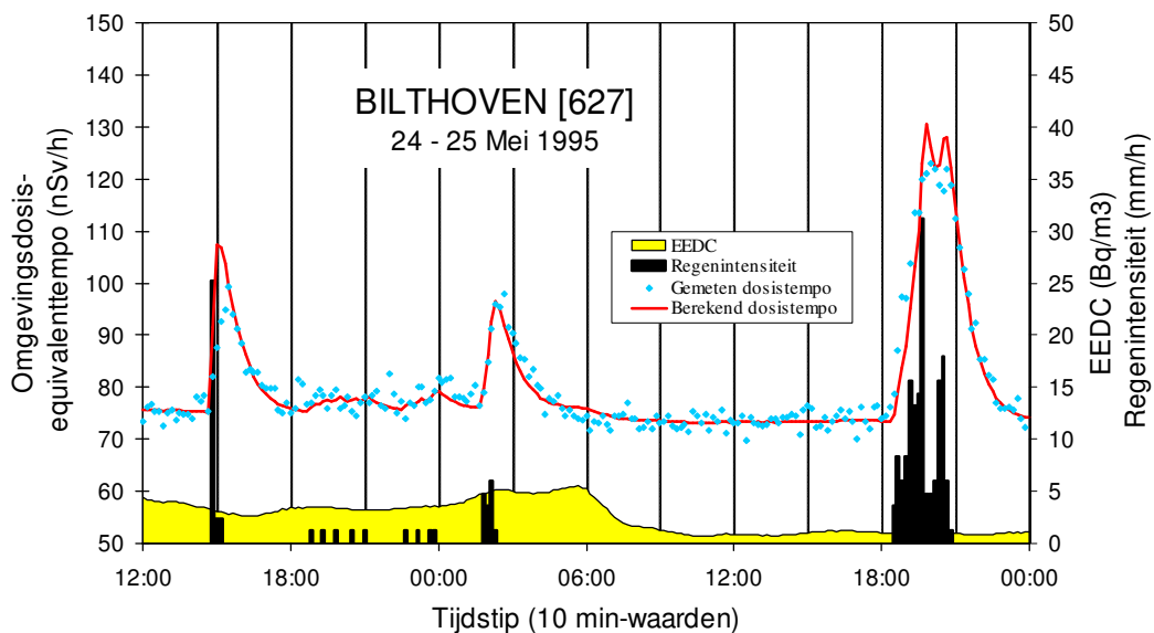
Figuur 2 Tien-minuutwaarden van het gemeten en het berekende omgevingsdosis-equivalenttempo, uitgezet tegen de op dezelfde lokatie gemeten regenintensiteit en de EEDC [Sme96; Sme97a]
