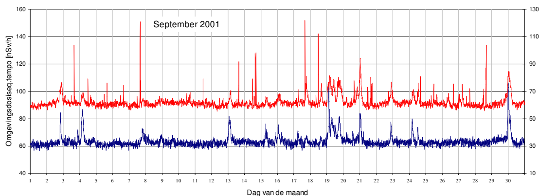
Figuur 10 Gemeten waarden van het omgevingsdosis-equivalent tempo op NMR-lokatie Petten (1006) (boven, rode lijn, rechteras) en de berekende waarden voor de natuurlijke achtergrond (beneden, blauwe lijn, linkeras). Aan de berekende waarden is op synthetische wijze 'telruis' toegevoegd.
