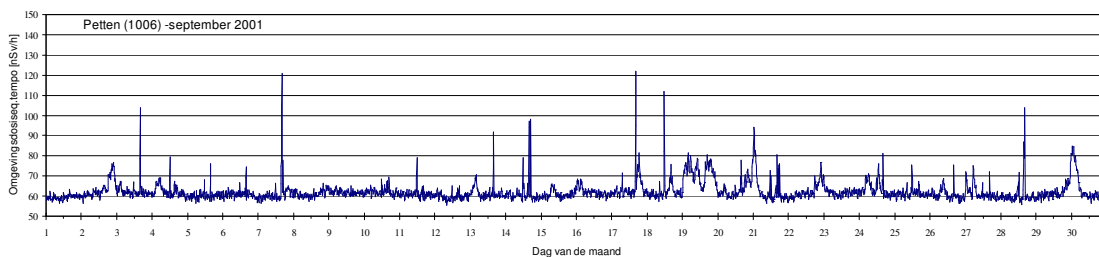
Figuur 7 Tien-minuutwaarden van het omgevingsdosisequivalenttempo, bepaald gedurende september 2001 op NMR-lokatie Petten (1006). Merk op dat de y-as loopt van 50-150 nSv/h, zodat variaties in de data sterk worden uitvergroot.
