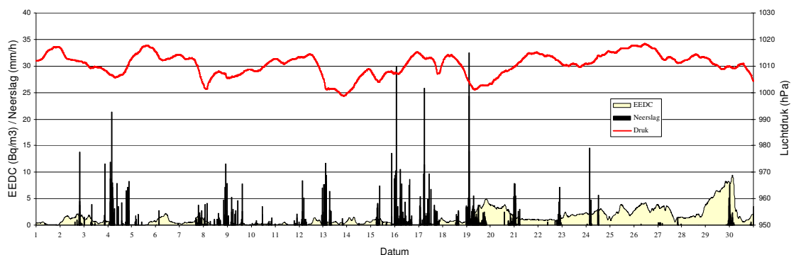
Figuur 8 Tien-minuutwaarden van luchtdruk en neerslag, bepaald gedurende september 2001 op KNMI-lokatie Amsterdam-Schiphol, en EEDC-data van NMR-lokatie De Zilk (444)
