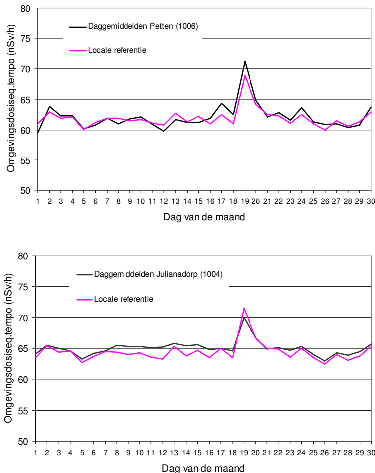
Figuur 11 Dagwaarden van het omgevingsdosissequivalenttempo van meetpost Petten (1006) (boven) respectievelijk Julianadorp (1004) (onder). In elke grafiek is tevens de volgens de MONET-methode bepaalde lokale referentiewaarde weergegeven.
