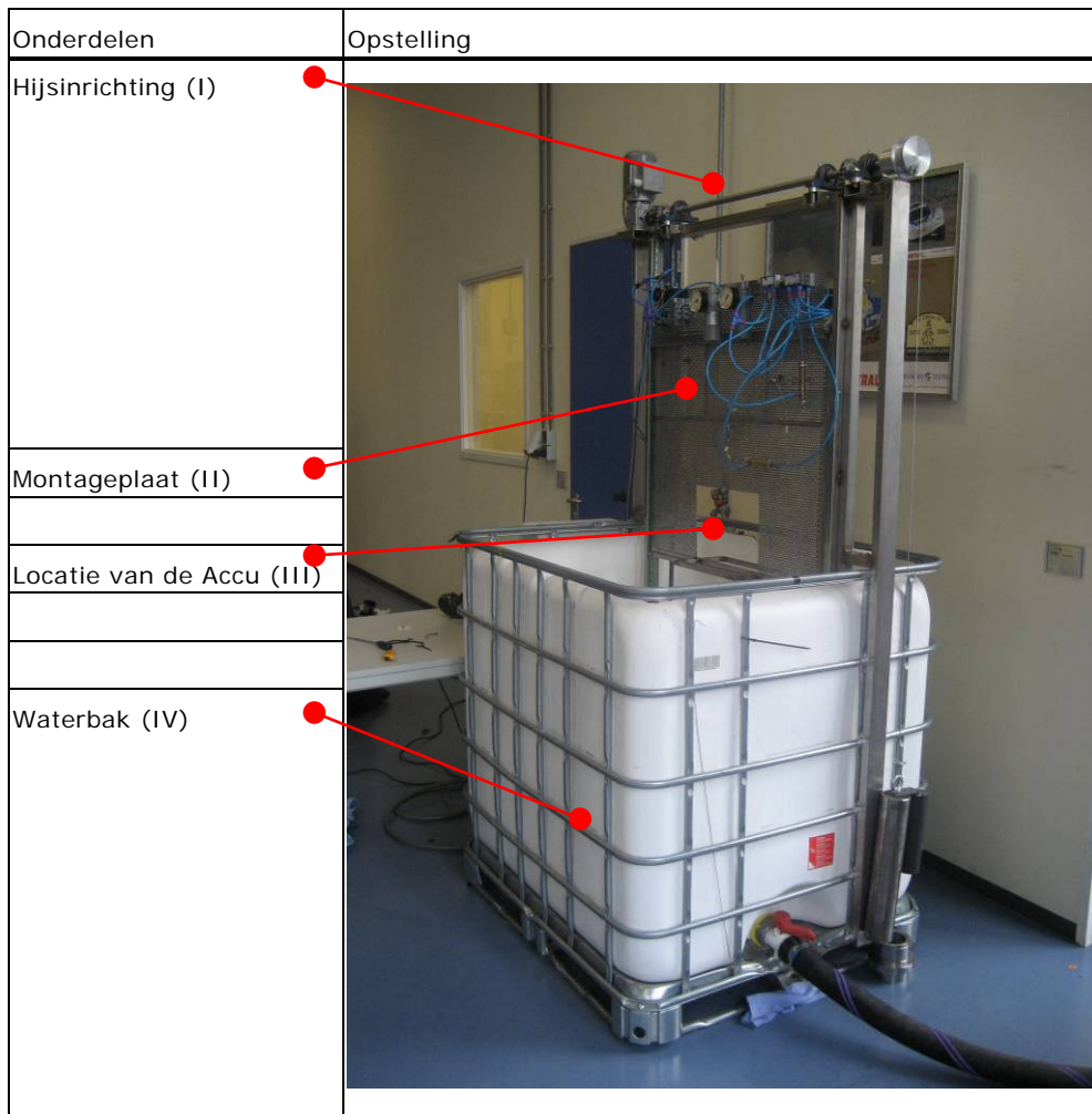
Figuur 3-1 Overzicht van de testopstelling
