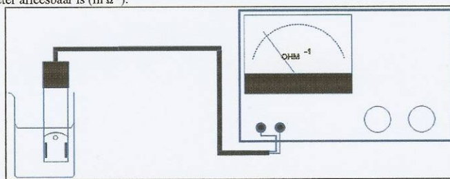
Figuur B.I-2 Een conductometer waarop een geleidbaarheidscel is aangesloten.
