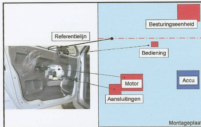
Figuur 2-1 Portier versus Montageplaat; positie van de testenonderdelen
