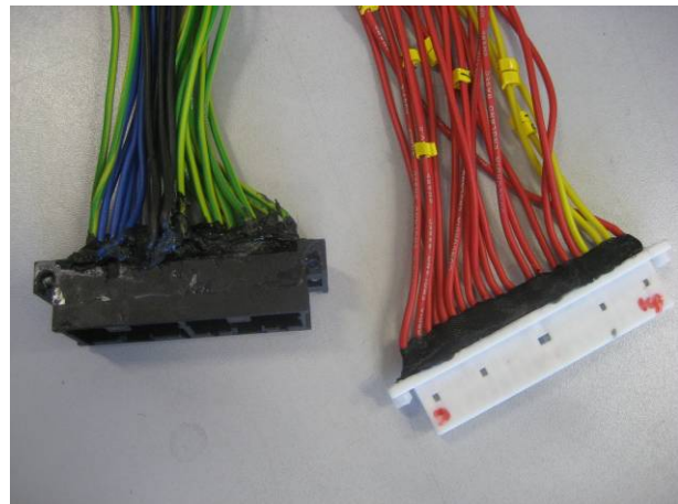
Figuur 3.4-5 Waterdichte aansluitingen
