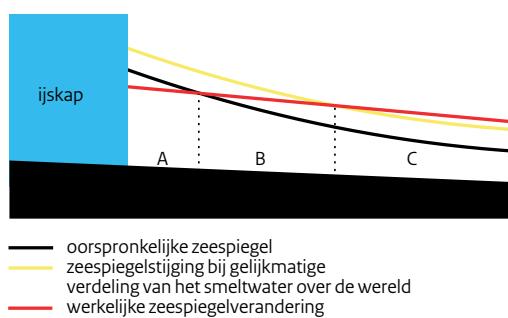
figuur 9. Illustratie van het effect van zelf-gravitatie op de lokale zeespiegel bij afkalving van een ijskap. In gebied A treedt zeespiegeldaling op; in B is de zeespiegelstijging kleiner dan de stijging bij een gelijkmatige verdeling; in C is de zeespiegelstijging groter dan bij een gelijkmatige verdeling.
