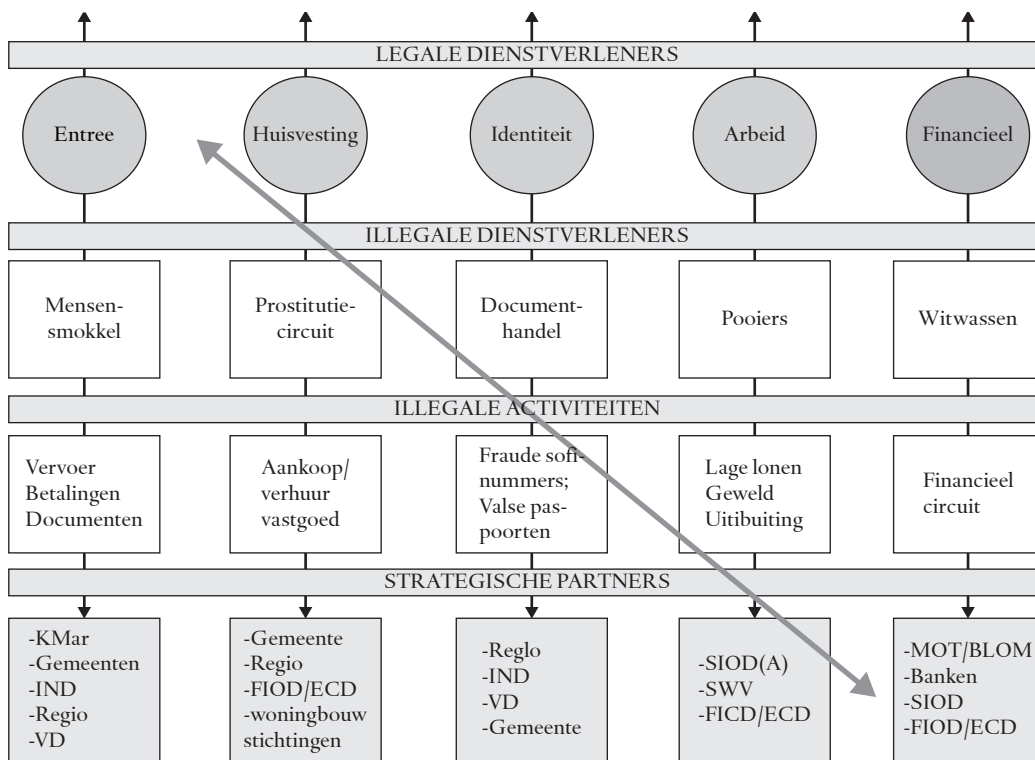
Figuur 10.1 Barrièremodel
