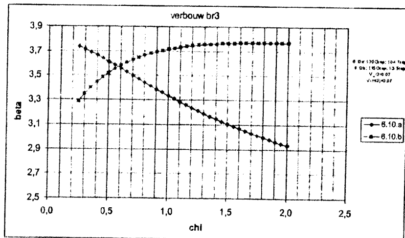
Figuur B1.1, Betrouwbaarheidsindex verbouw CC3 bij voorgestelde verificatieregels.
