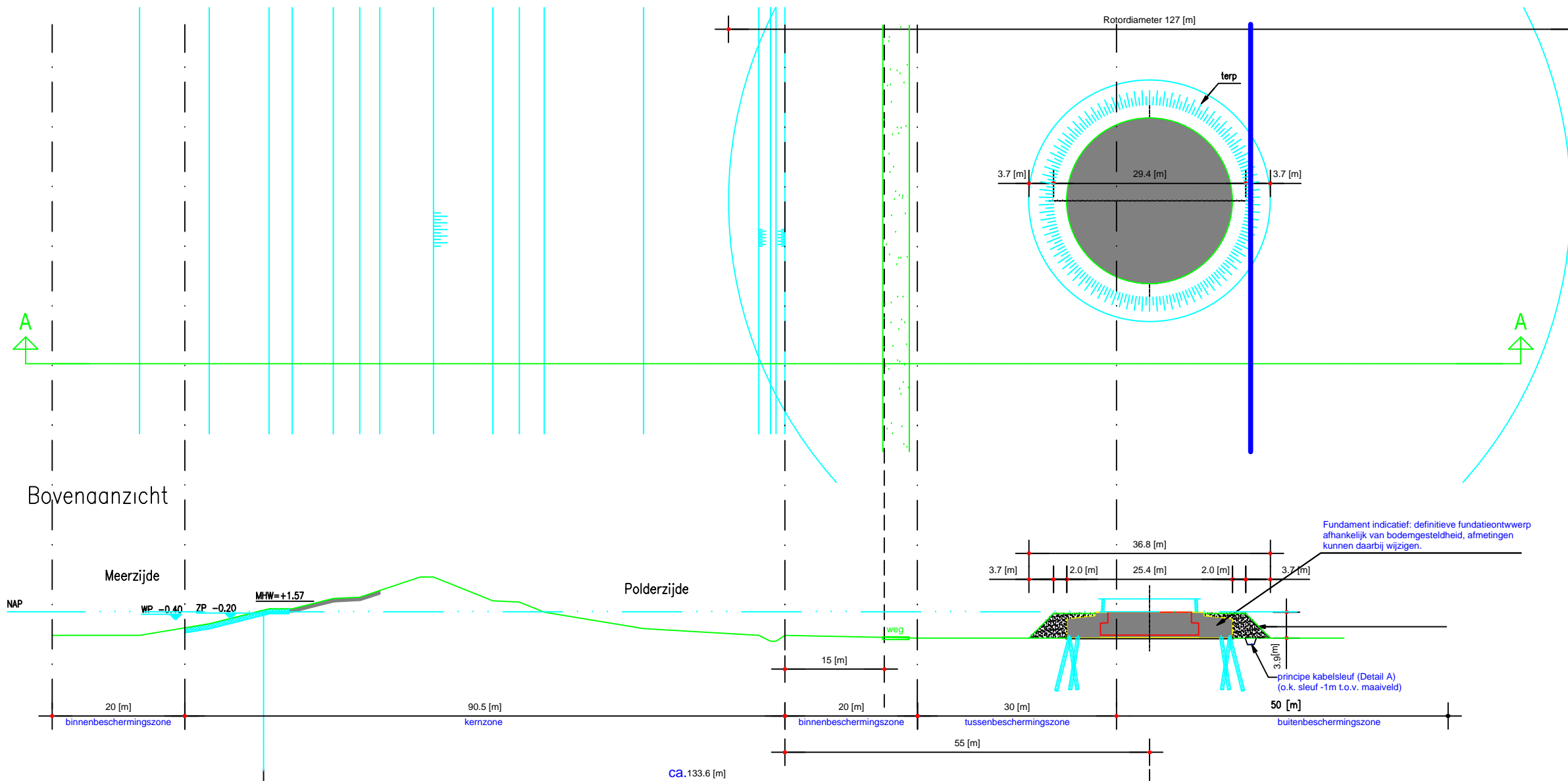
Dwarsprofiel kilometerpaal 17,40
