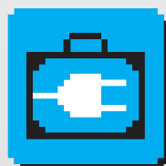
Electronisch Zakendoen
