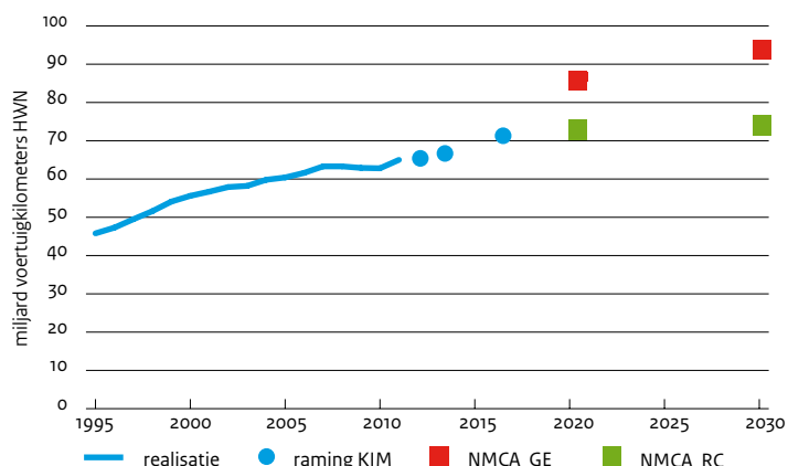
Figuur 3.12 Ontwikkeling van het wegverkeer op het hoofdwegennet. Bron: ministerie IenM.
