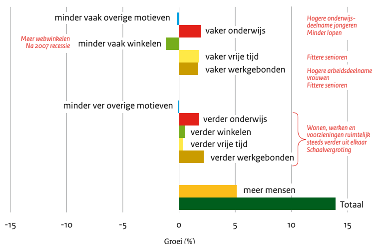
Figuur 2.11 Opbouw van de ontwikkeling van het fietsgebruik tussen 2000 en 2011. Bron: KiM op basis van OVG/MON/OViN.
