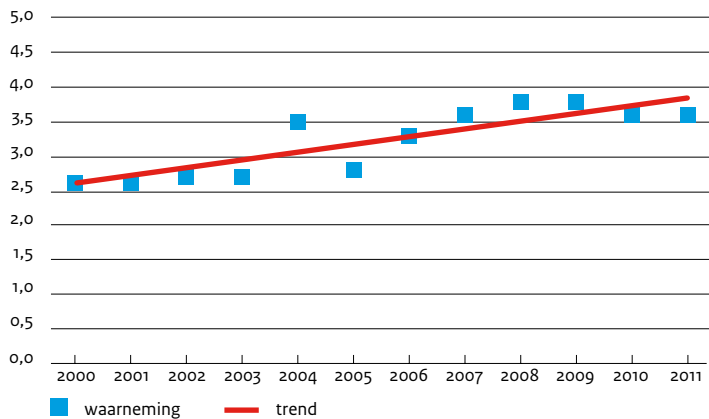
Figuur 2.9 Aandeel (in procenten) van fietsritten die onderdeel zijn van een treinverplaatsing ten opzichte van het totaal aantal fietsritten Bron: OVG/MON/OViN, bewerking KIM.
