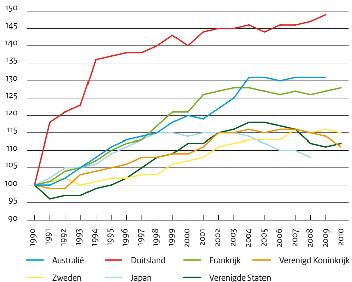
Figuur 3.4 Reizigerskilometers auto en 'light trucks', 1990–2009. Index: 1990=100. Bron: ITF (2012).
