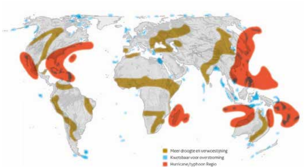
Figuur 14 Gevolgen van klimaatveranderingen wereldwijd (Ministerie van Defensie, 2010)
