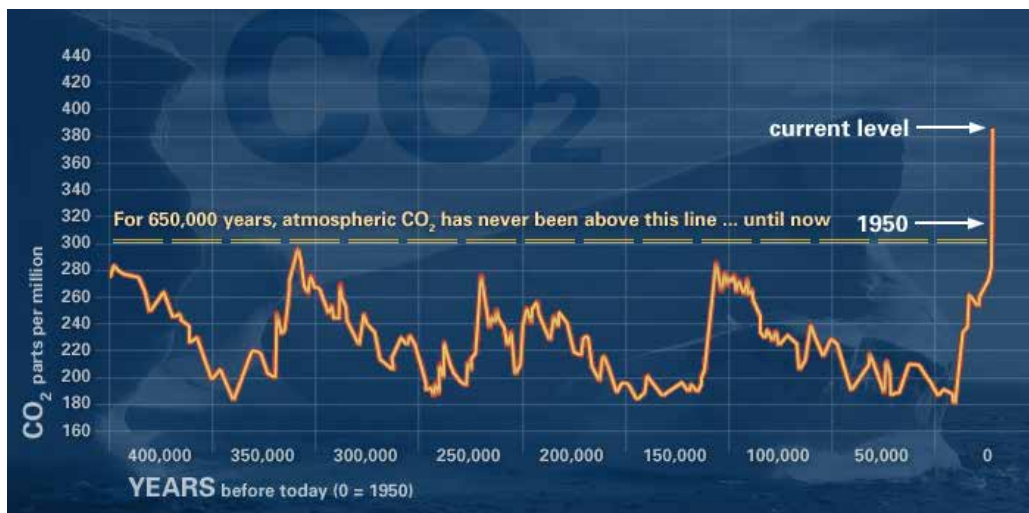
Figuur 13 In de afgelopen vijftig jaar is de hoeveelheid CO 2 in de atmosfeer enorm toegenomen (NASA)
