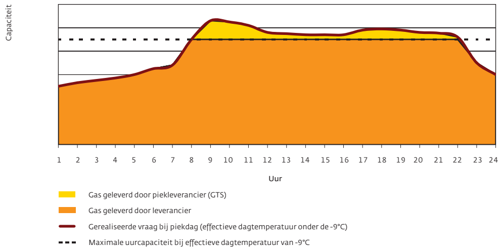
Figuur 11: Algemene werking van de pieklevering
