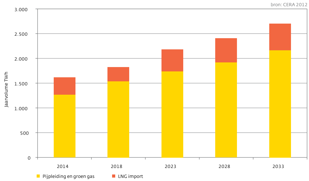
Figuur 3: Benodigde import voor Noordwest-Europa
