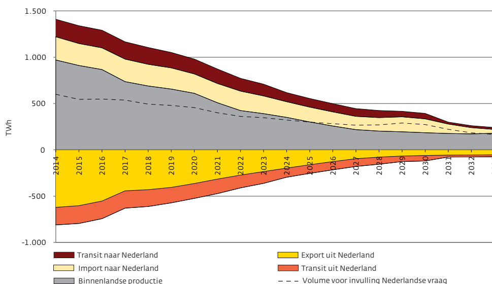
Figuur 6: Verwachtings scenario
