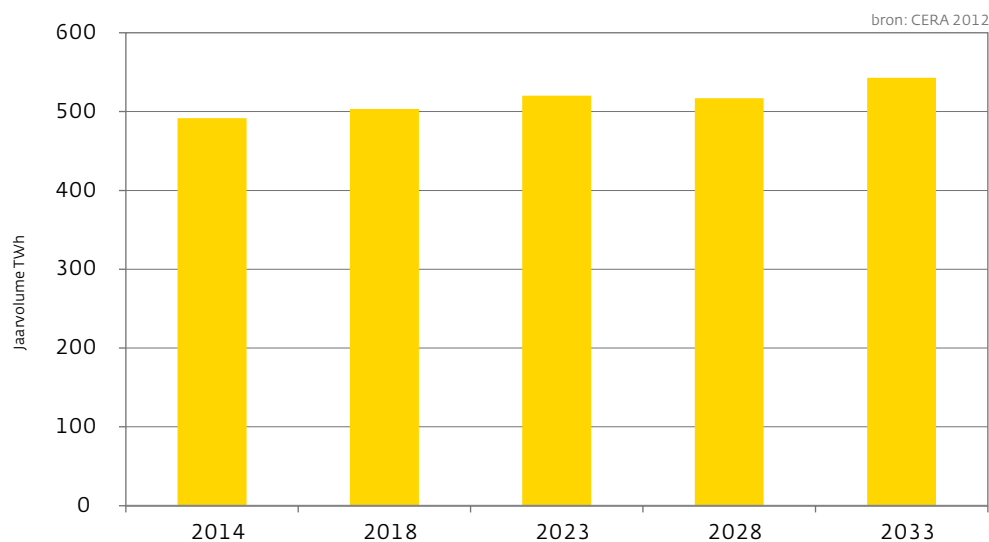
Figuur 4: Nederlandse gasvraag
