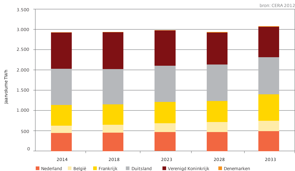
Figuur 1: Noordwest-Europese gasvraag
