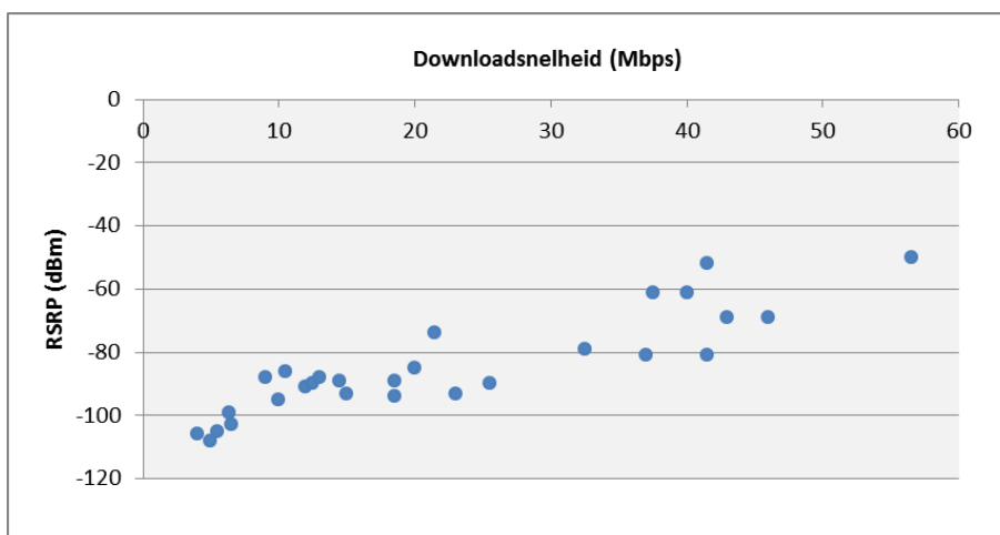
Figuur F.10: Strooidiagram van signaalsterkte (RSRP) en downloadsnelheid in 800 MHz band
