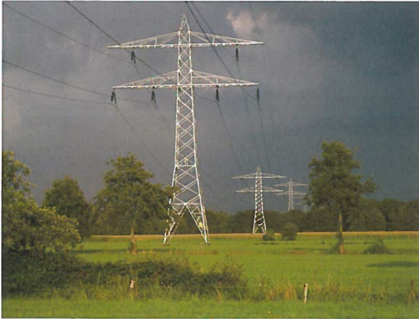
Figuur 2 Hoogspanningslijn Utrecht Lage Weide – Soest (locatie tussen mast 19 en mast 20, kijkend langs mast 20 in de richting van Soest)
