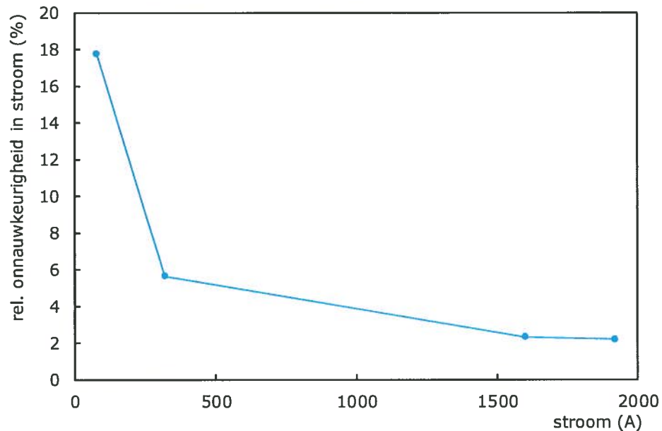
Figuur 17 Weergave van de relatieve meetonnauwkeurigheid in de circuitstroom van de 150 kV-lijn in Maartensdijk voor 5, 20, 100 en 120% van de nominale stroom (1600 A)
