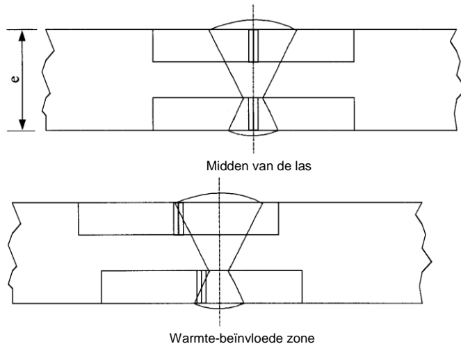
Warmte-beïnvloede zone
