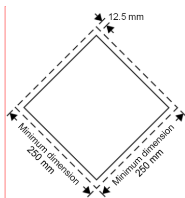
Groot etiket (behalve voor klasse 7)
