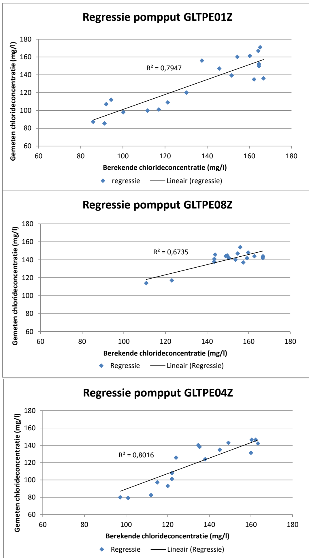
Figuur 24: Regressie tussen gemeten en berekende chlorideconcentraties in drie pompputten van Tiendweg
