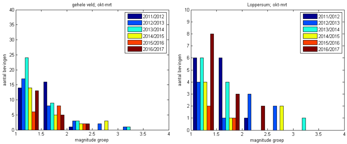
Figuur 2: Aantal aardbevingen ≥ 1,0 in de winter periode van het gasjaar (oktober t/m maart) voor links het gehele Groningen gasveld en rechts de regio rond Loppersum.
