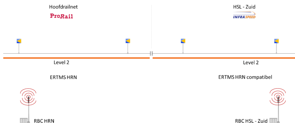
Figuur 5 Upgrade HSL-Zuid RBC tot compatibel met RBC HRN
