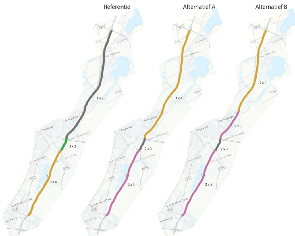
Figuur 3.2: Weergave aantal rijstroken op de hoofdrijbaan in de referentie en in de alternatieven A en B. Het aantal rijstroken op de parallelrijbaan (bij Leiden/Leiderdorp) is niet gevisualiseerd (dit wijzigt niet t.o.v. de referentie).
