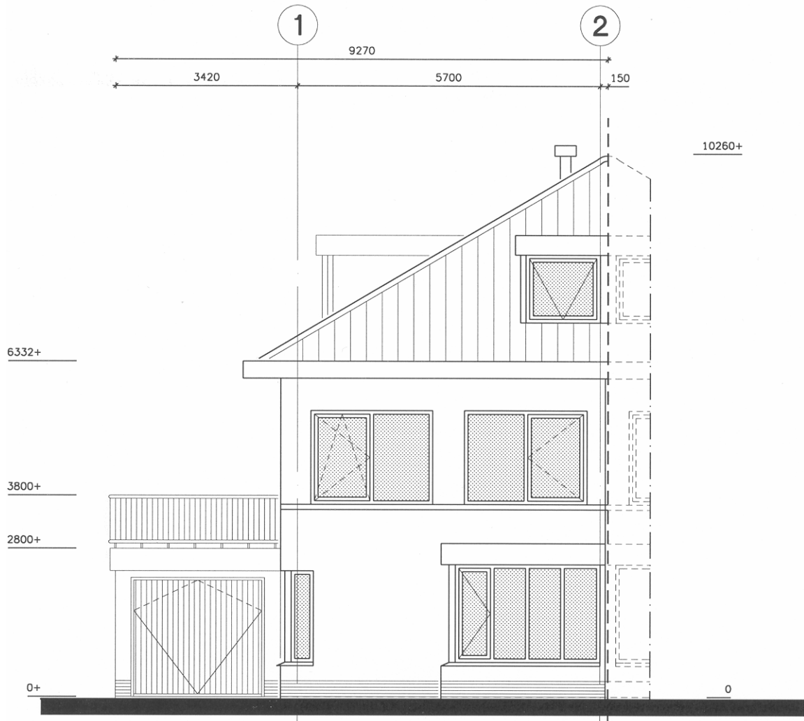
figuur 6.5 - Voorgevel van bouwplan 2 (schaal 1:100)
