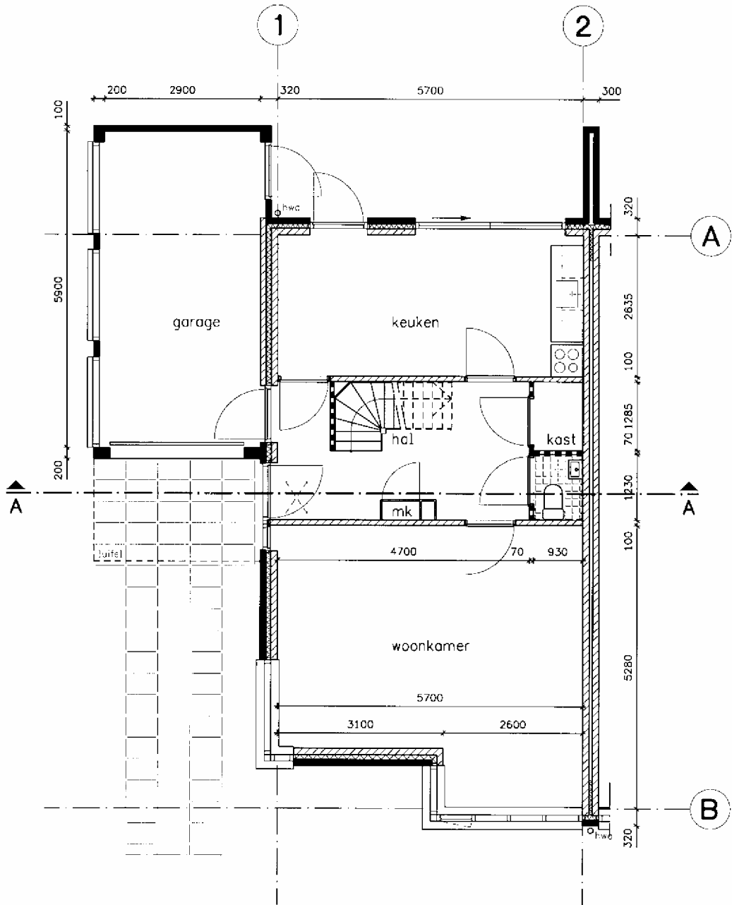
figuur 6.2 - Begane grond van bouwplan 1 (schaal 1:100)
