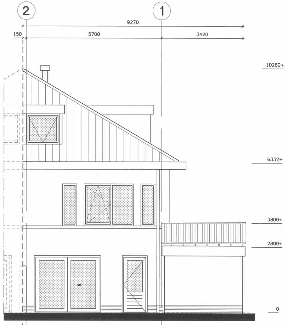
figuur 6.6 - Achtergevel van bouwplan 2 (schaal 1:100)
