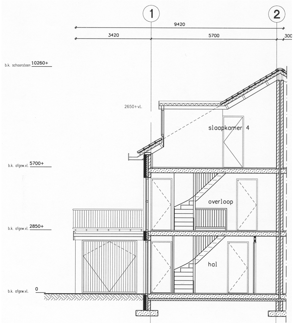
figuur 6.8 - Doorsnede van bouwplan 1 (schaal 1:100)
