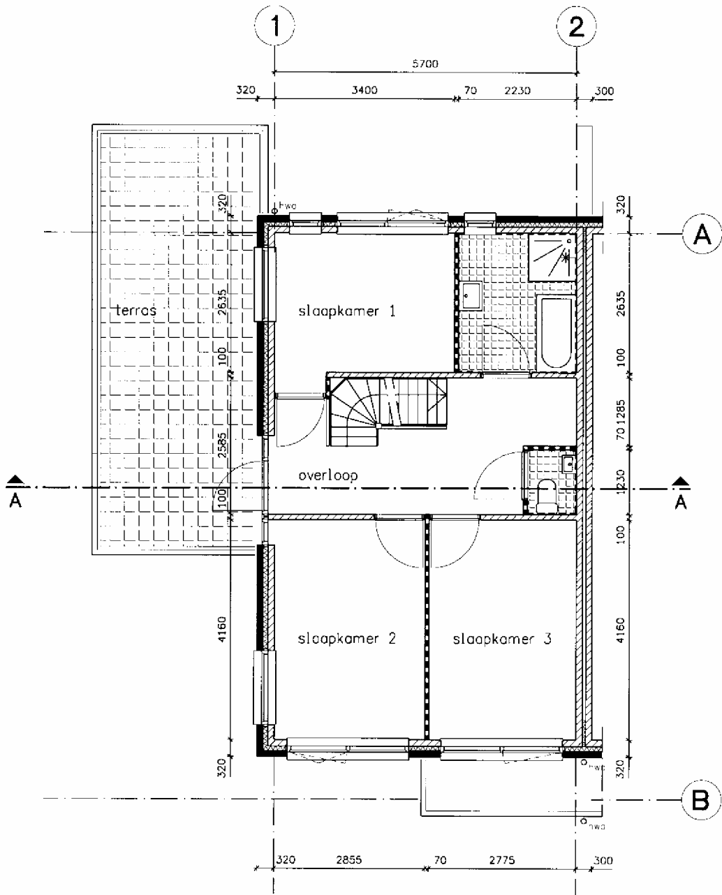
figuur 6.3 - Eerste verdieping van bouwplan 1 (schaal 1:100)
