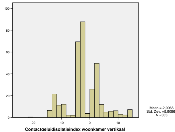
Figuur 6.11: Verdeling van de verticale contactgeluidisolatie in de woonkamer ( I_{co} in dB)
