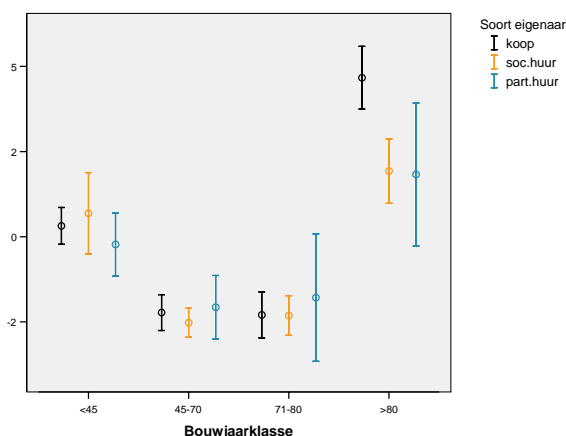
Figuur 6.6: Gemiddelde luchtgeluidisolatie slaapkamer horizontaal
