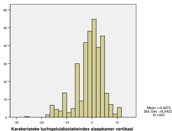
Figuur 6.4: Verdeling van de verticale luchtgeluidisolatie in de (hoofd)slaapkamer ( I_{lu,k} in dB)
