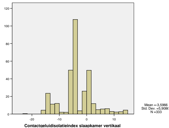
Figuur 6.12: Verdeling van de verticale contactgeluidisolatie in de (hoofd)slaapkamer ( I_{co} in dB)
