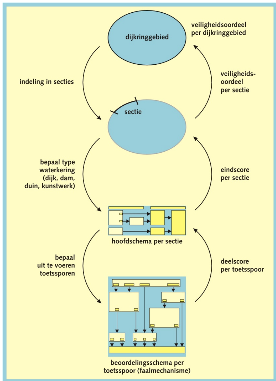
Figuur 2 - 2.1 Beoordelingswijze voor primaire waterkeringen
