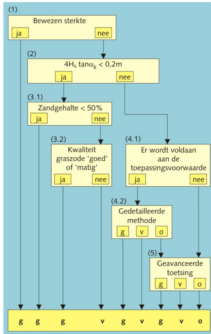
Figuur 8 - 4.5 Beoordelingsschema Erosie door golfklap GEKL
