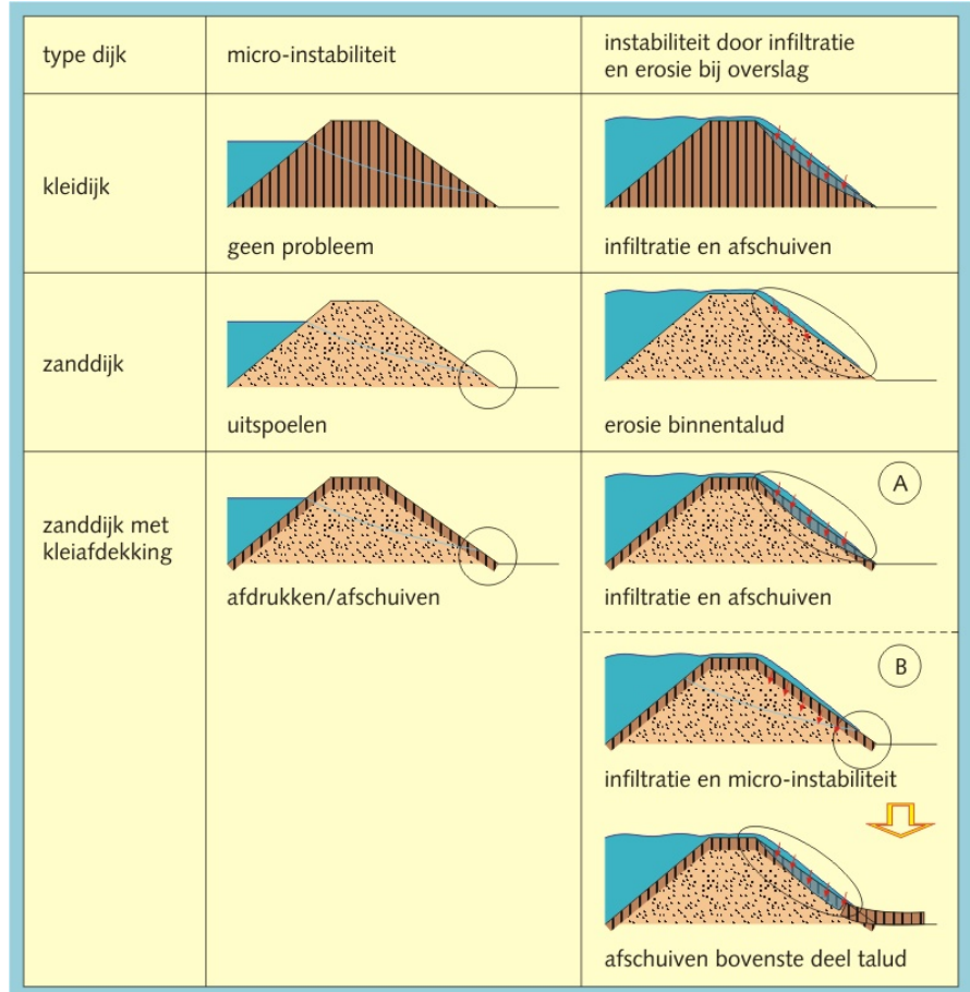
Figuur 5 - 1.2 Micro-instabiliteit en instabiliteit door infiltratie en erosie bij overslag
