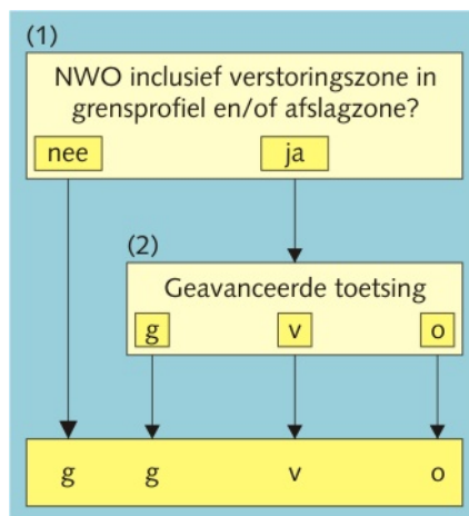
Figuur 6 - 4.6 Beoordelingsschema Niet-waterkerende objecten NWO
