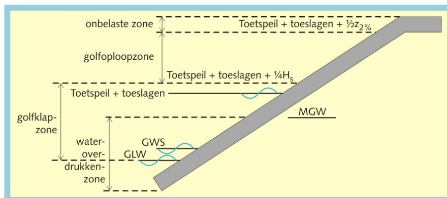
Figuur 8 - 3.2 Schematische weergave van de belastingzones op het talud
