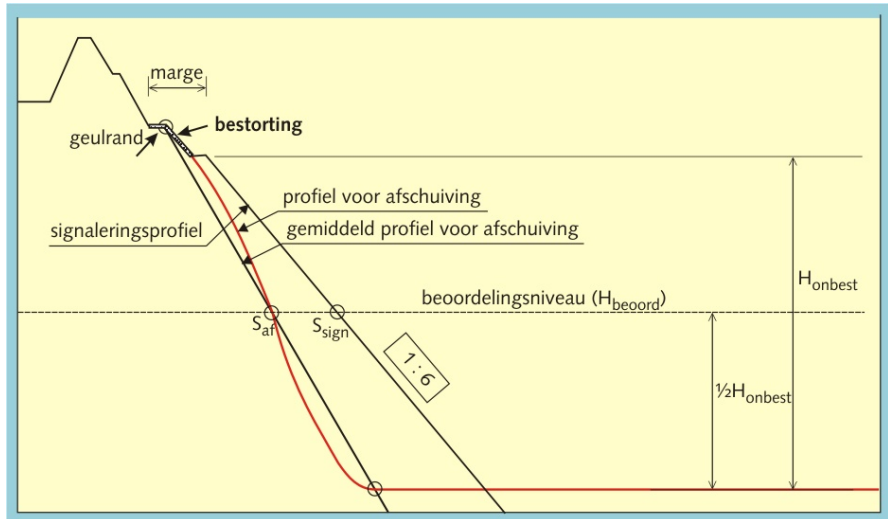
Figuur 9 - B2.2 Signaleringsprofiel afschuiving bestorte oever
