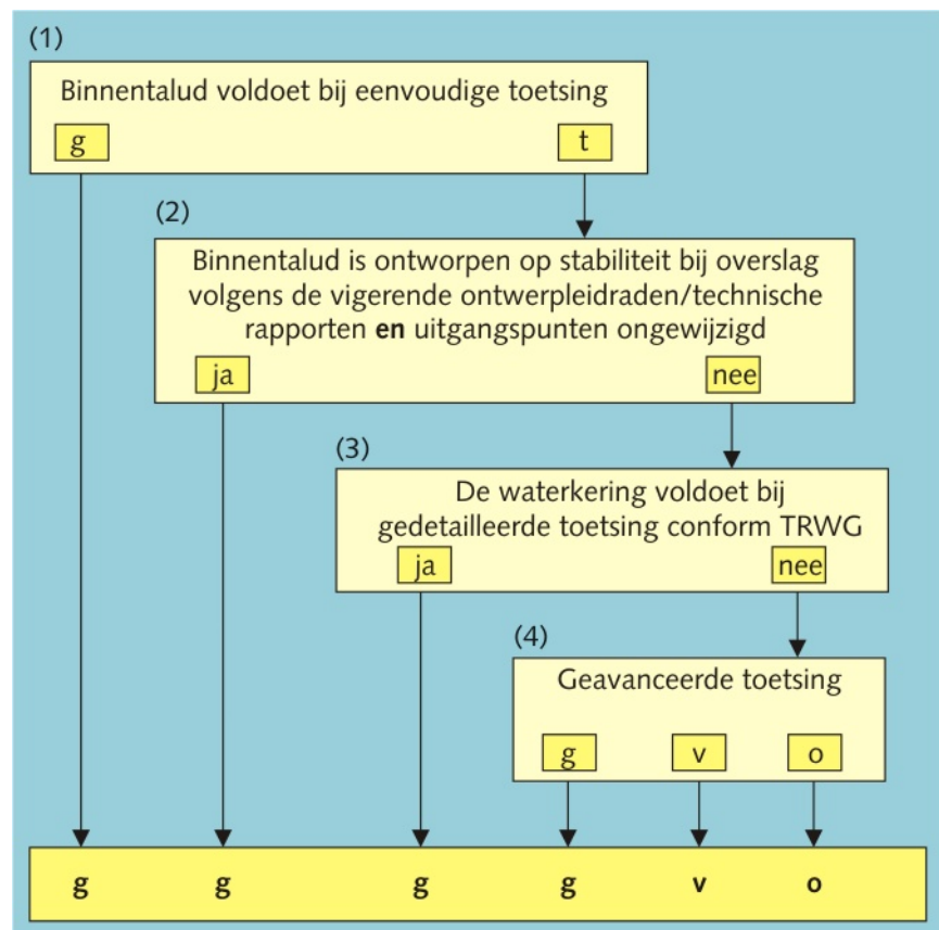
Figuur 8 - 4.9 Beoordelingsschema Afschuiving GAF voor het binnentalud
