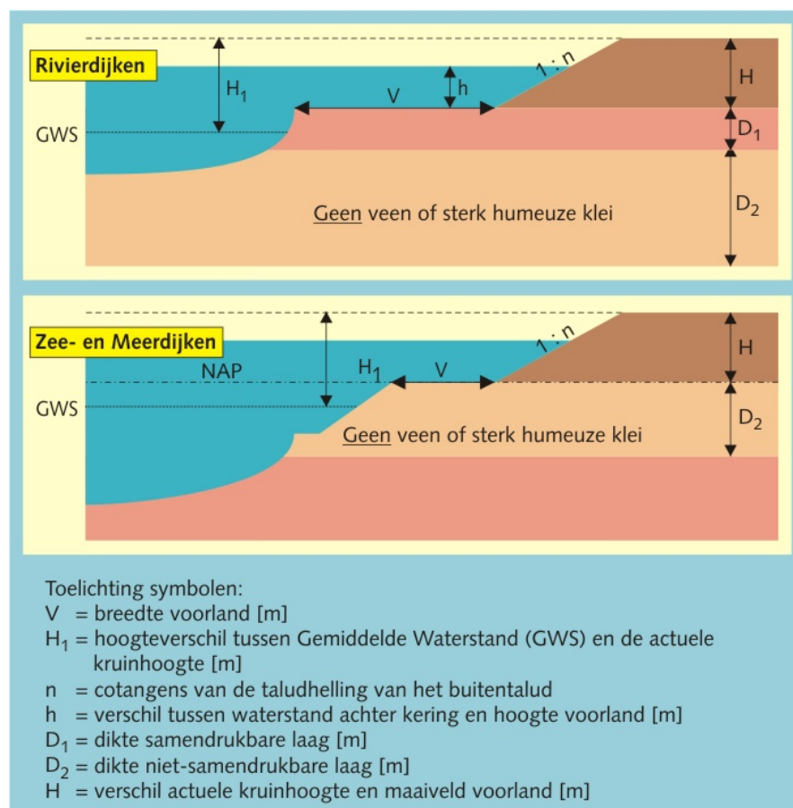
Figuur 5 - 4.17 Geometrische toets Macrostabieleit buitenwaarts
