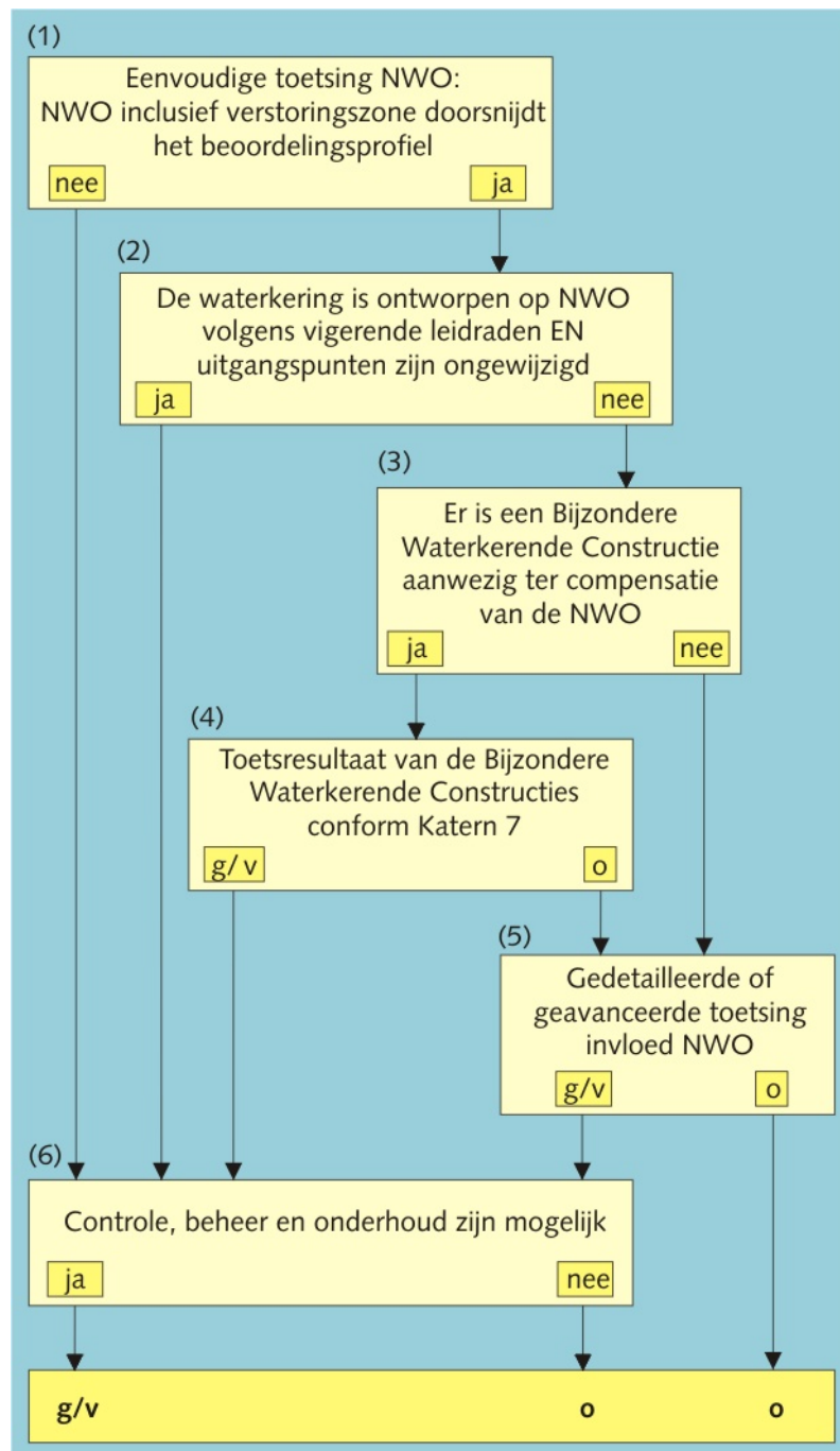
Figuur 10- 4.1 Beoordelingsschema niet-waterkerende objecten
