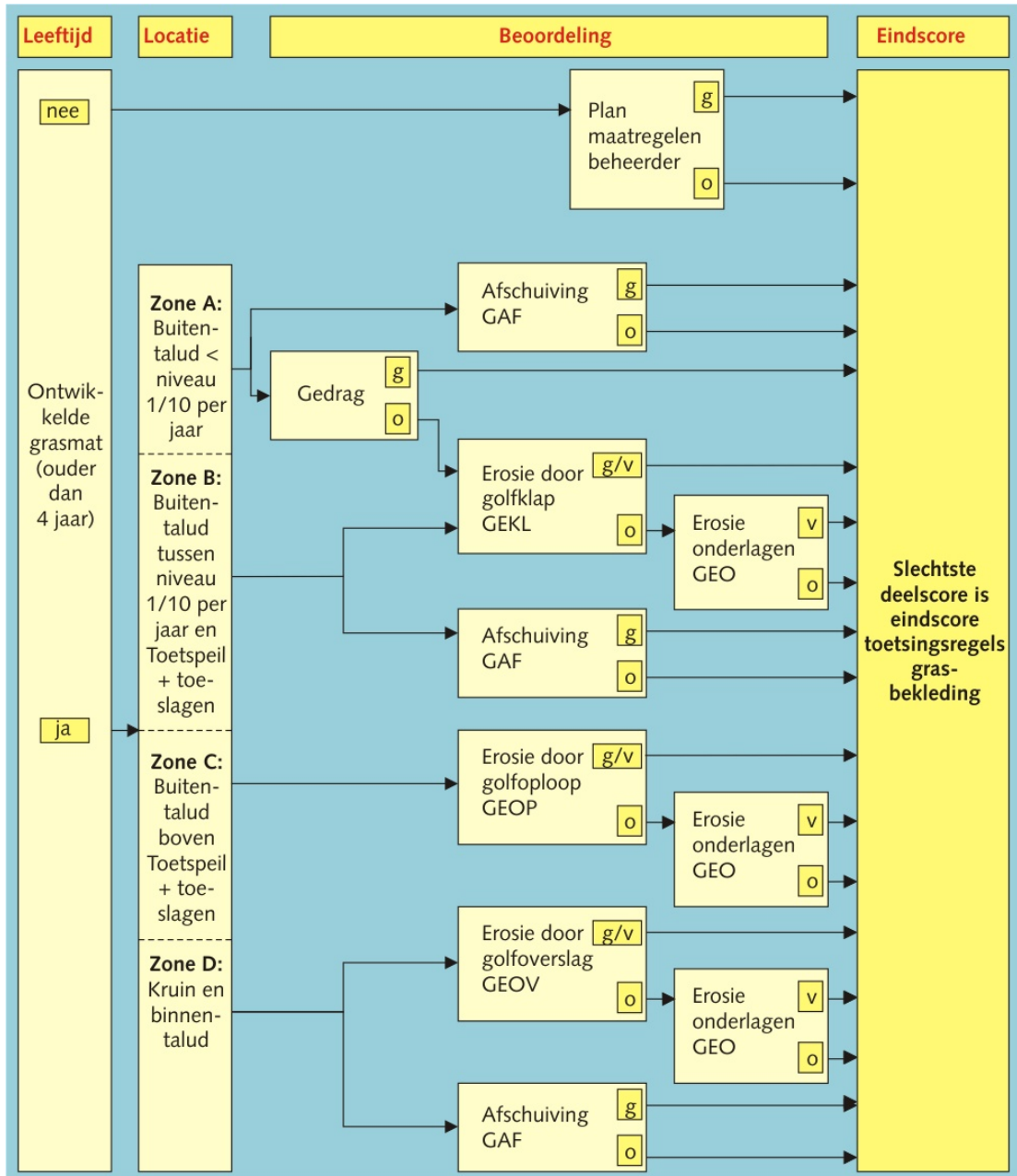
Figuur 8 - 4.2 Hoofdschema toetsing grasbekleding
