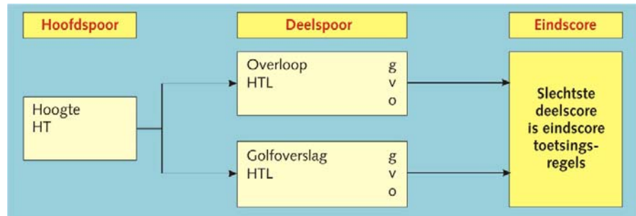
Figuur 5 - 4.2 Hoofdschema voor de beoordeling van de Hoogte HT van Maaskaden
