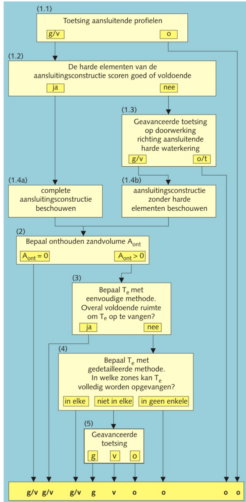
Figuur 6 - 4.7 Beoordelingsschema aansluitingsconstructies
