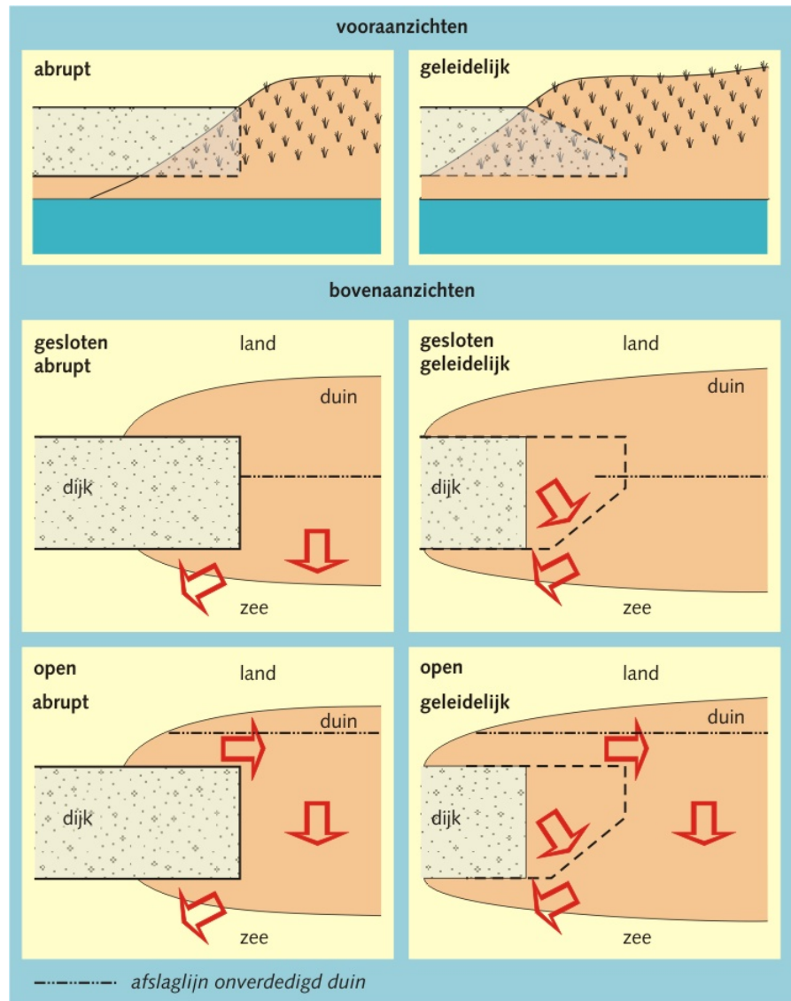
Figuur 6 - 1.2 Principevoorbeelden aansluitingsconstructies Type I
