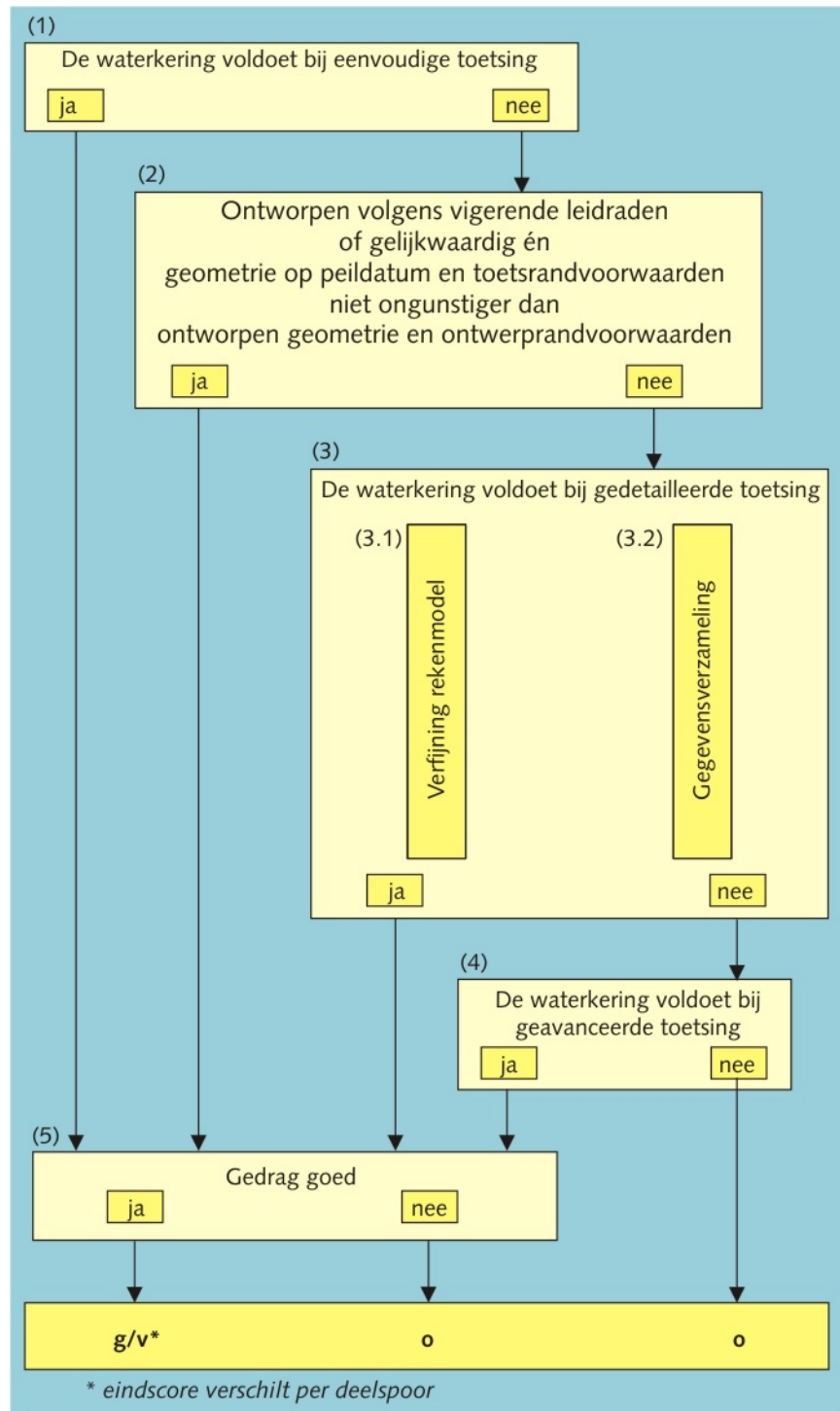
Figuur 5 - 4.5 Beoordelingsschema stabiliteit voor dijken en dammen (STPH, STBI, STBU en STM)
