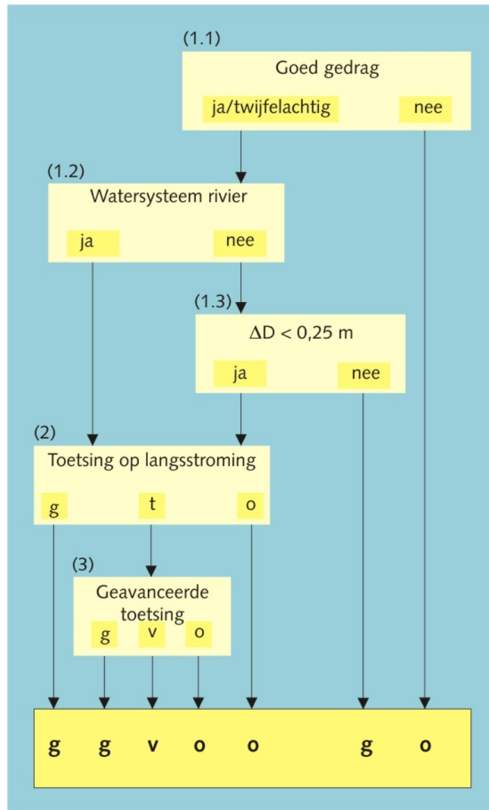
Figuur 8 - 2.8 Beoordelingsschema Toplaaginstabiliteit onder langsstroming ZTS
