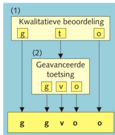
Figuur 8 - 3.21 Beoordelingsschema Overgangsconstructies bij asfaltbekledingen AOC
