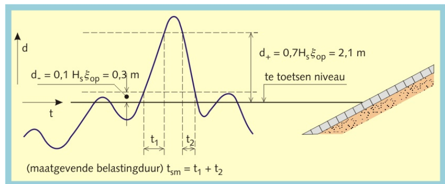
Figuur 8 - 2.2 Voorbeeld bepalen maatgevende belastingduur t_{sm}
