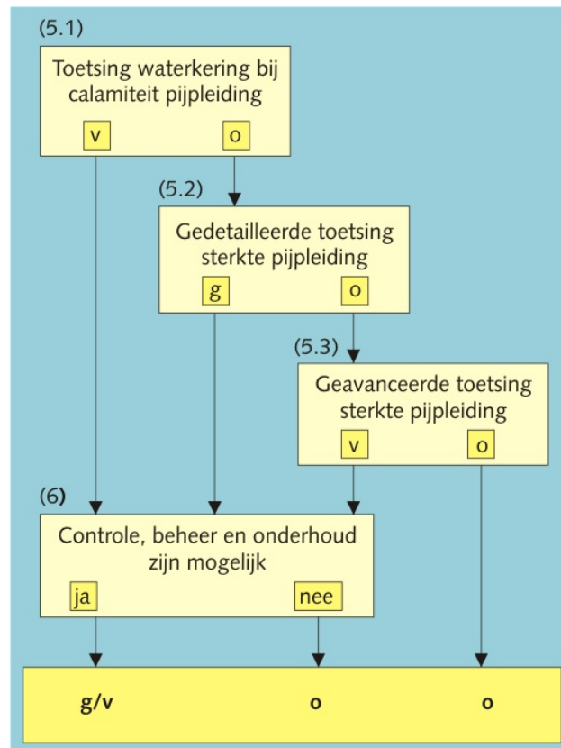
Figuur 10 - 4.2 Uitwerking stap 5 voor toetsing van pijpleidingen
