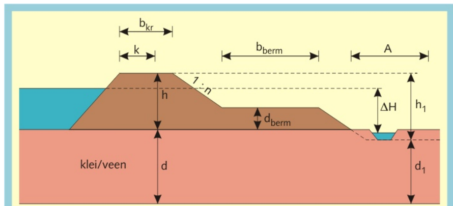
Figuur 5 - 4.12 Geometrische toets Macrostabiteit binnenwaarts voor profiel met berm
