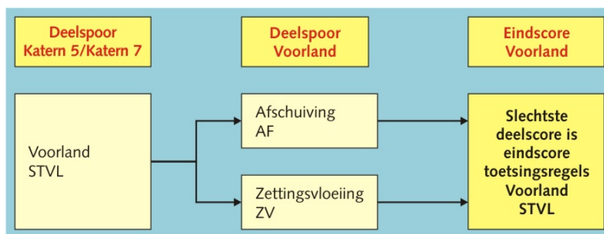
Figuur 9 - 2.1 Hoofdschema toetsing Stabiliteit Voorland STVL
