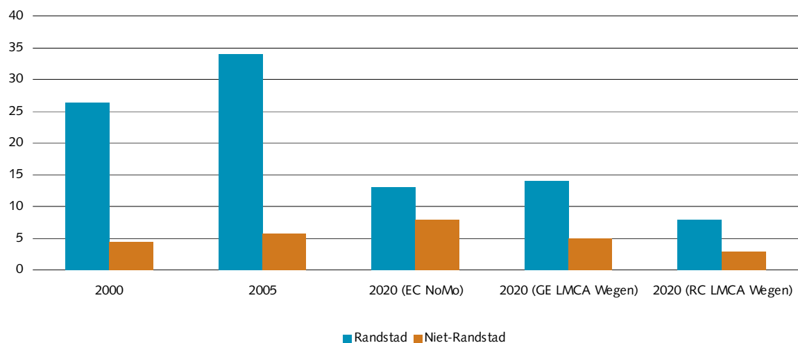
Figuur 3.4 Ontwikkeling voertuigverliesuren in files op het hoofdwegennet per scenario, naar landsdelen, in miljoenen Bron: RWS-DVS
