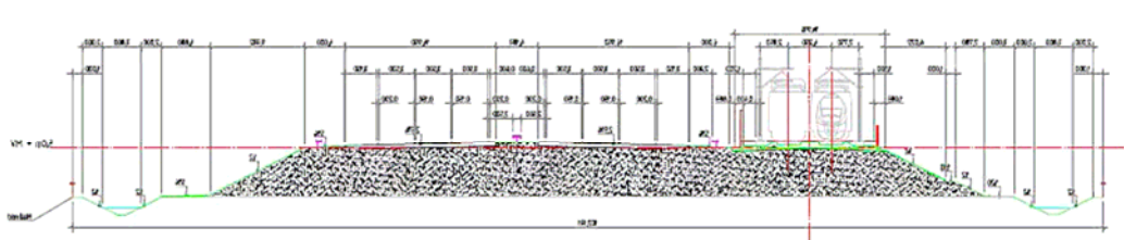
Dwarsprofiel spoorlijn en A27 separaat, gelijktijdig aangelegd
