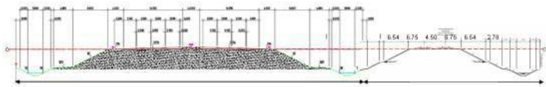
Dwarsprofiel uitgaande van separate ligging
