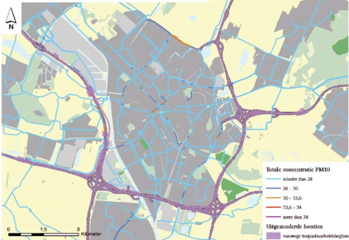
Utrecht, concentratie PM10 in 2011 na lokaal beleid
