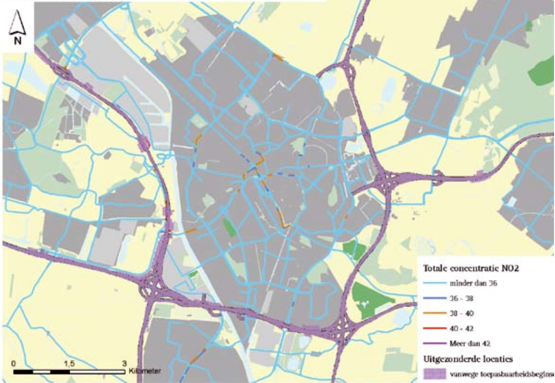
Utrecht, concentratie NO2 in 2015 na lokaal beleid
