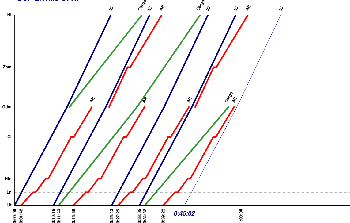
Grafiek 6.1: Grafische weergave baanvakbelastingen ERTMS Level 2.
