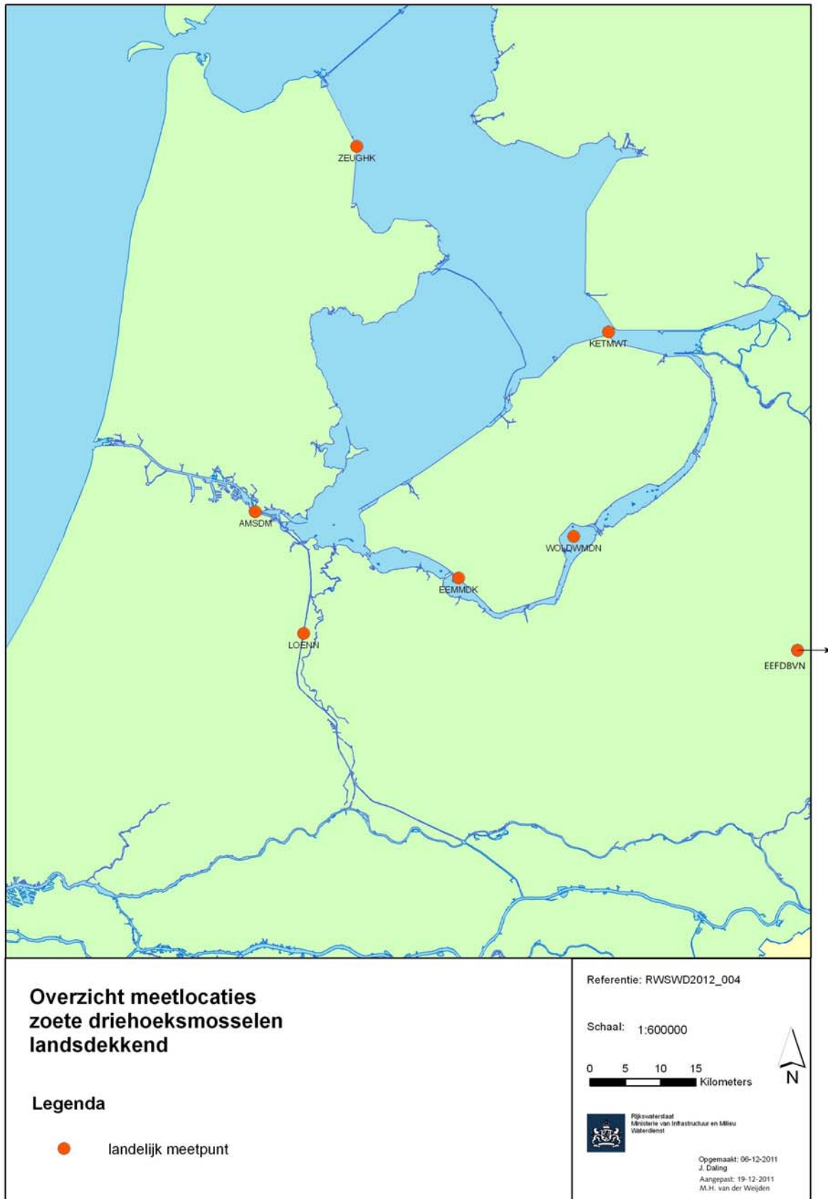
Figuur 2. Overzicht meetlocaties zoete driehoeksmosselen landsdekkend
