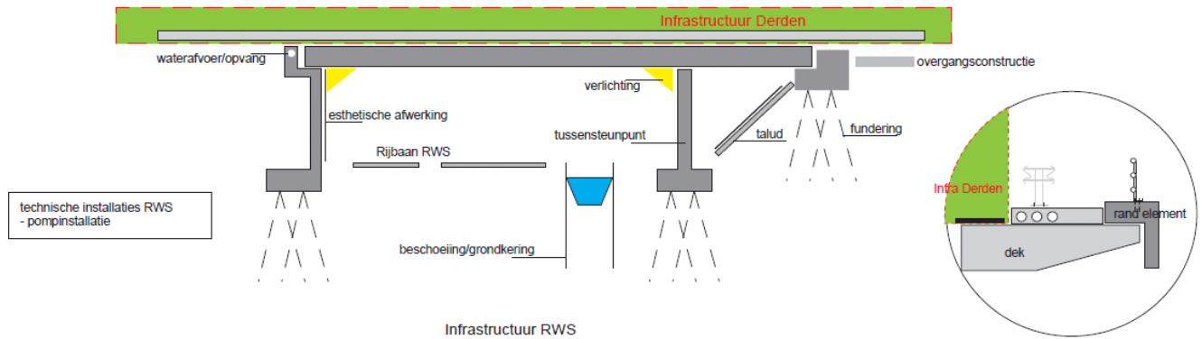
Figuur 3: Systemdefinitie
