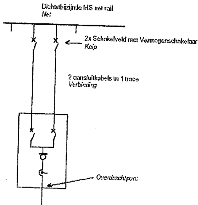
Figuur 6 MS aansluiting op MS net rail ( 3 - 10 MVA )
