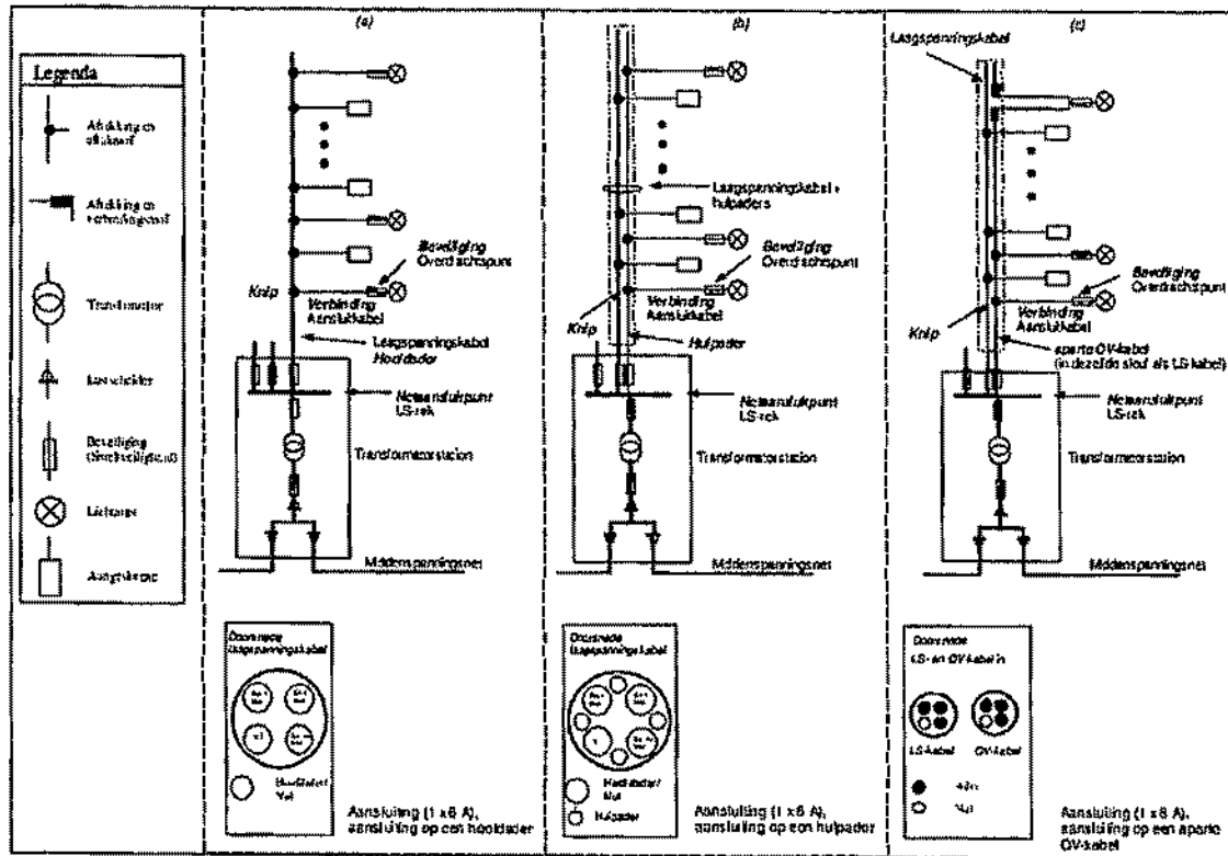
Figuur 1 LS geschakeld aansluitingen (1*6A)
