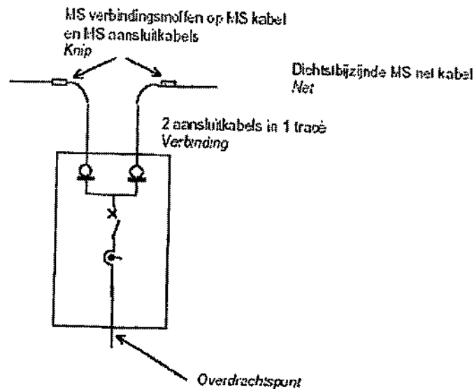
Figuur 4 Zuivere MS aansluiting ( 0,3 – 3 MVA )
