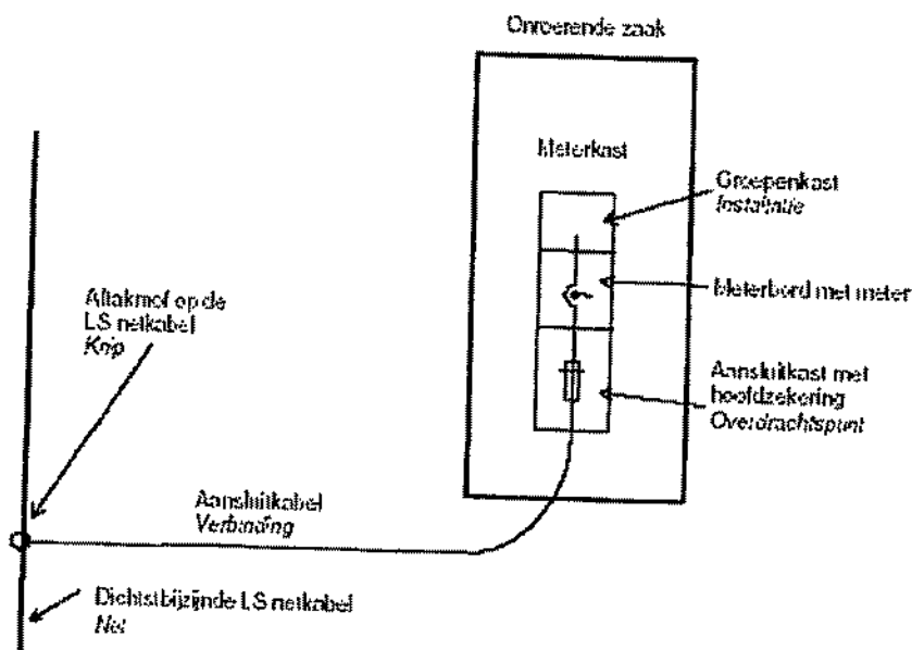
Figuur 2 LS aansluiting (3* 25 A – 60 kVA)
