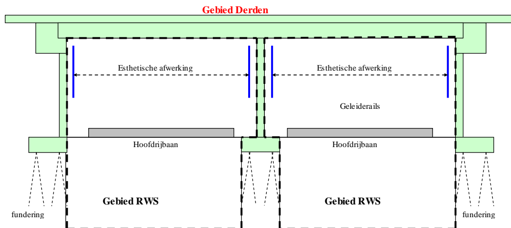
Figuur 1: Principe begrenzing van een viaduct
