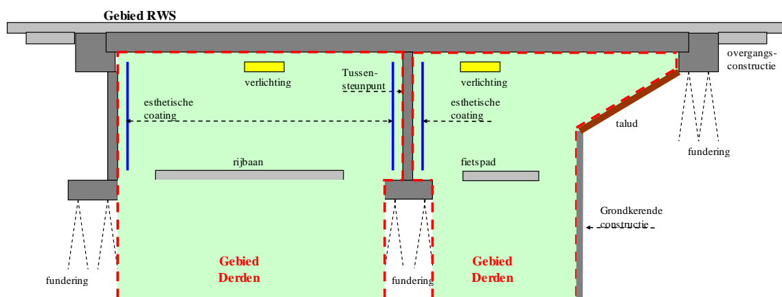
Figuur 2: Principe begrenzing van een viaduct
