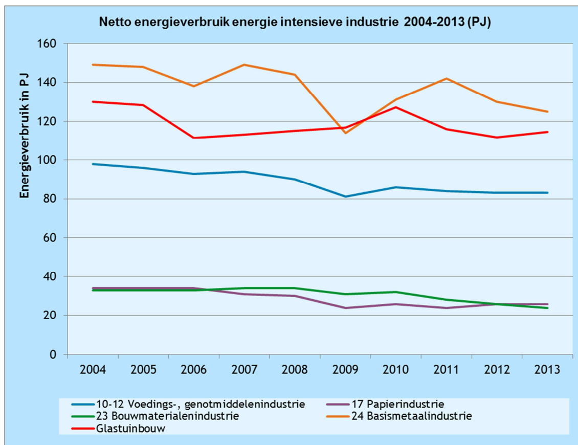
Figuur 5.2: Netto energiegebruik energie-intensieve industrie (2004-2013)
