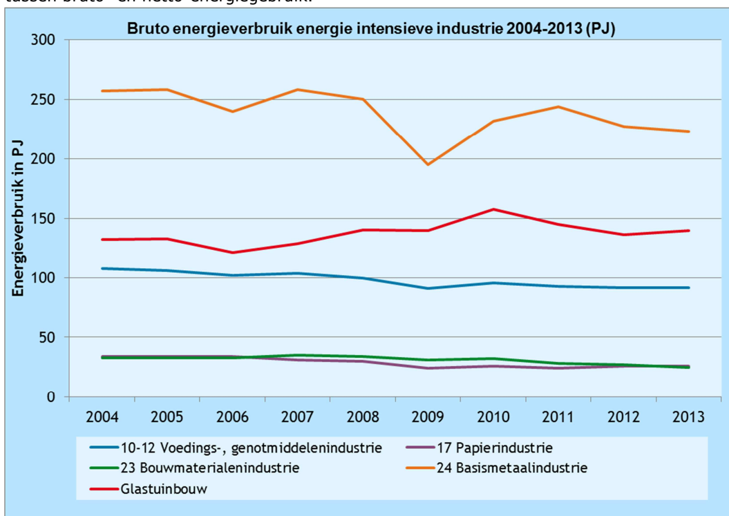
Figuur 5.1: Bruto energiegebruik energie-intensieve industrie (2004-2013) Bron: CBS Statline (industrie) en LEI (glastuinbouw)
