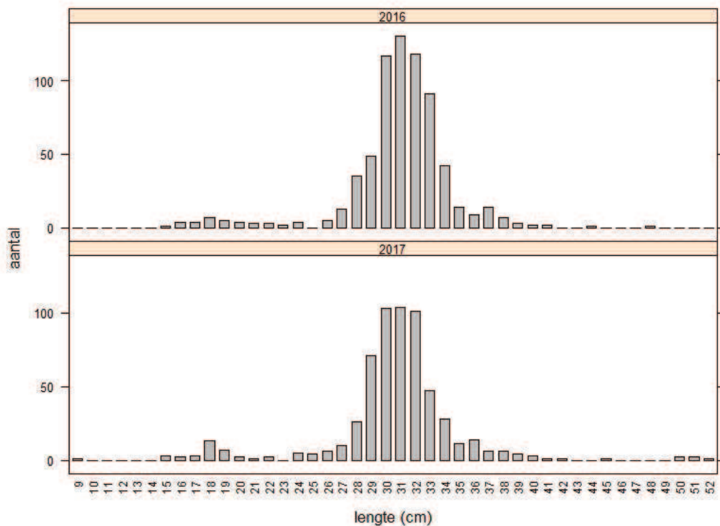
Figuur 3.5 Lengteopbouw van de commerciële baarsvangsten met standwantnetten 101 mm, bemonsterd in de marktmonitoring in september-december van 2016 en 2017. Baars mag worden aangeland vanaf 22 cm.
