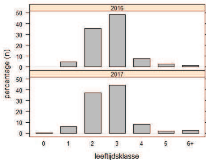
Figuur 3.6 Geschatte leeftijdsopbouw van de commerciële baarsvangsten met standwantnetten 101 mm, bemonsterd in de marktmonitoring in september-december van 2016 en 2017. De y-as geeft het geschatte percentage van het totaal aantal vissen weer.
