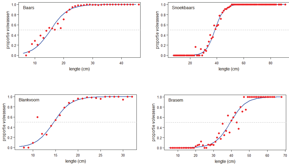
Figuur B.2.1 De gemiddelde proportie vis die volwassen (paarijpp) is per lengteklasse.
