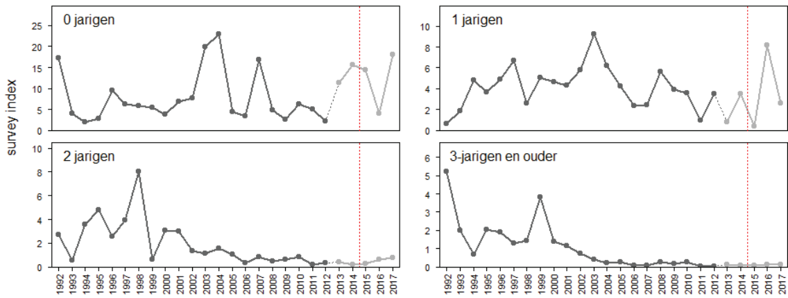
Figuur 3.3 Biomassa-index voor baars, opgesplitst in leeftijden. Trend voor het IJsselmeer en Markermeer gecombineerd. De biomassa-index betreft de gemiddelde biomassa-dichtheid (kg per hectare) van de openwatersurvey (kuil/boomkor en elektrokor survey in de verhouding 0.7:0.3). De rode lijn is de start van het nieuwe visserijbeheer. Van 2012 op 2013 is in de kuil/boomkor survey gewisseld van tuig, van grote kuil naar verhoogde boomkor.
