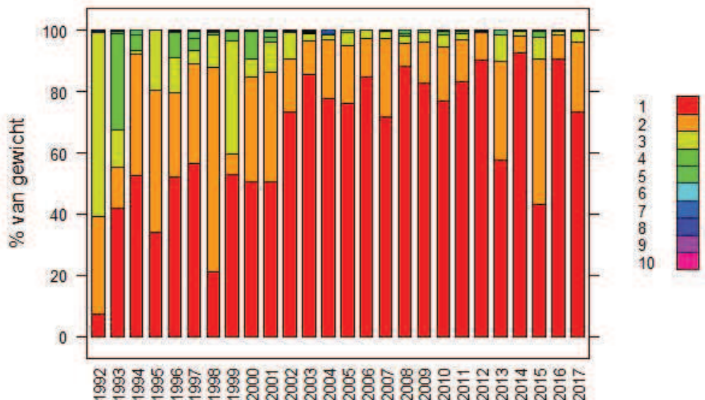
Figuur 3.4 Leeftijdopbouw van baars (zonder de 0-jarige) gevangen in de openwatersurvey met de kuil/boomkor en de elektrokor door de jaren heen. Het percentage van het gewicht per leeftijdsklasse. Van 2012 op 2013 is gewisseld van tuig, van grote kuil naar verhoogde boomkor.
