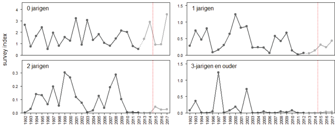
Figuur 4.3 Biomassa-index voor snoekbaars, opgesplitst in leeftijden. Trend voor het IJsselmeer en Markermeer gecombineerd. De biomassa-index betreft de gemiddelde biomassa-dichtheid (kg per hectare) van de openwatersurvey (kuil/boomkor en elektrokor survey in de verhouding 0.7:0.3). De rode lijn is de start van het visserijbeheer. Van 2012 op 2013 is in de kuil/boomkor survey gewisseld van tuig, van grote kuil naar verhoogde boomkor.
