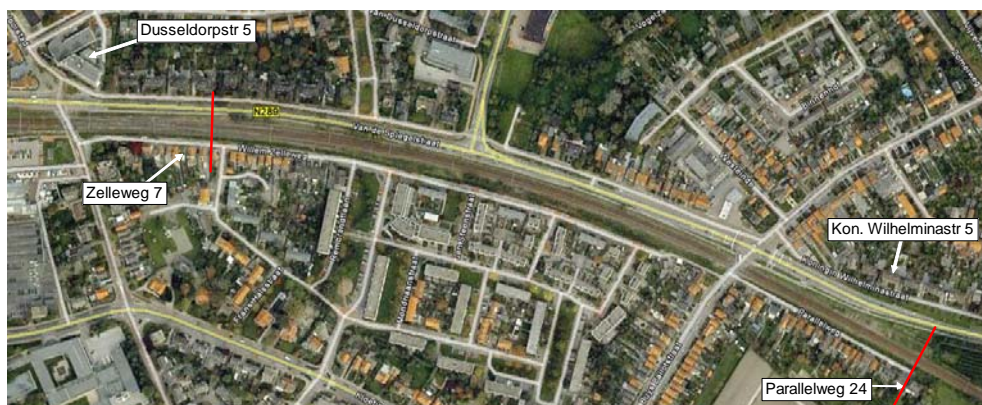
Figuur 2: Overzicht langdurige meting. Naast de referentiepanen (van Dusseldorpstraat en Koningin Wilhelminastraat) zijn de twee locaties weergegeven waar treinpassages zijn opgenomen (rode lijnen).
