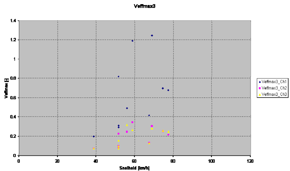
Figuur 25: Trillingsniveau tegen treinsnelheid bij referentiepand 3 (voor Captrein België passages in de meetperiode).
