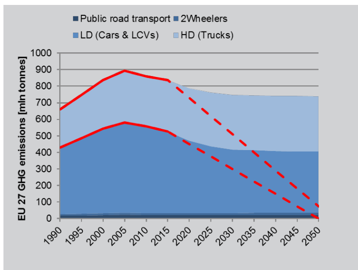
Figuur 1: Verwachte Europese emissies broeikasgas wegverkeer per vervoersmodus op basis van staand beleid (blauwe vlakken) en benodigde reducties voor het halen van de Parijs-doelstelling (rode lijnen)
