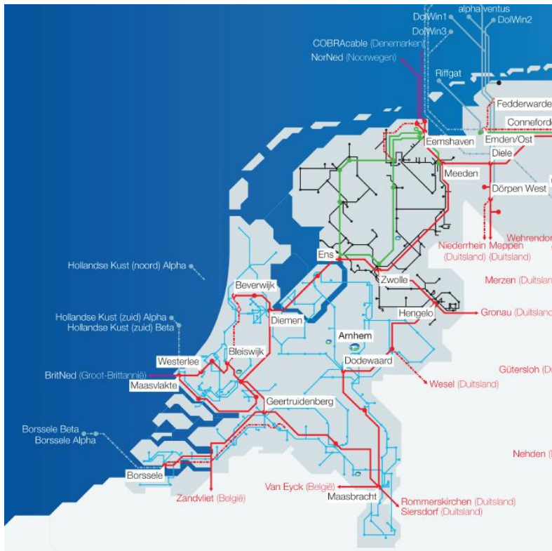
Figuur 4.18 – Transmissienetwerk en interconnectoren (Bron: TenneT)
