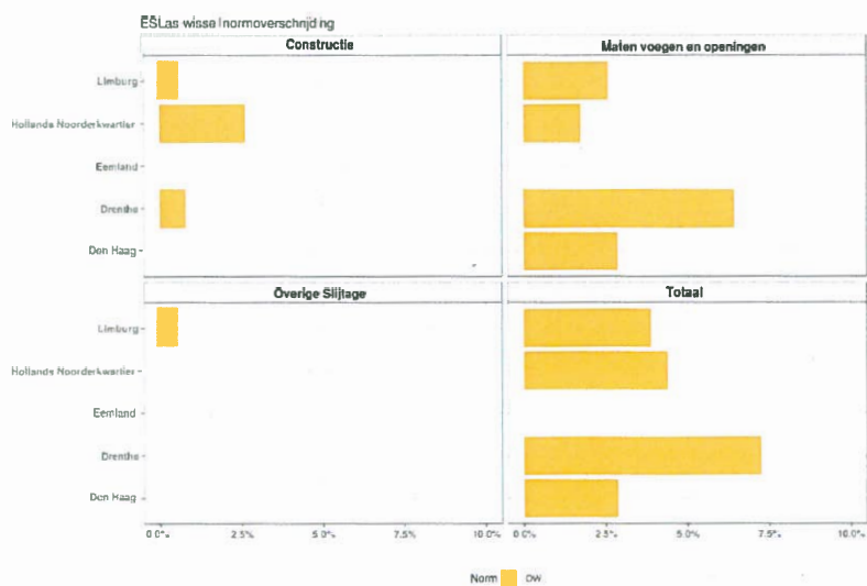
Figuur 6. Het percentage normoverschrijdingen bij het object ESLas-wissel voor de vijf contractgebieden uitgesplitst naar het aspect van de geconstateerde bevinding. Het totaal is de som van de geconstateerde normoverschrijdingen over alle aspecten.
