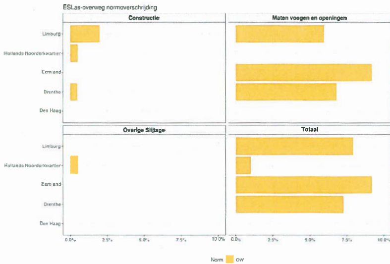
Figuur 7. Het percentage normoverschrijdingen bij het object ES-lasoverweg voor de vijf contractgebieden uitgesplitst naar het aspect van de geconstateerde bevinding. Het totaal is de som van de geconstateerde normoverschrijdingen over alle aspecten
