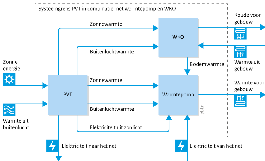
PVT: Gecombineerde elektriciteits- en warmteopwekking met zonnepanelen
