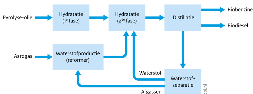
Figuur 10.3 Opwaarderding pyrolyse-olie met geïntegreerde waterstofproductie
