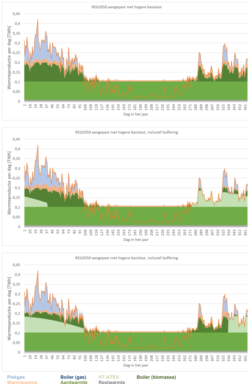
Figuur 6.3. Warmteproductieprofiel voor warmtenetten in het aangepaste REG2050-scenario met hogere basislast, zoals in de tekst beschreven. Boven: aangepaste scenario zonder buffering bij aantreden koude maanden. Midden: inclusief HT-ATES, start productie bij aantreden koude maanden. Onder: inclusief HT-ATES, start productie 2 maanden verschoven. De rode lijn geeft het verbruik weer
