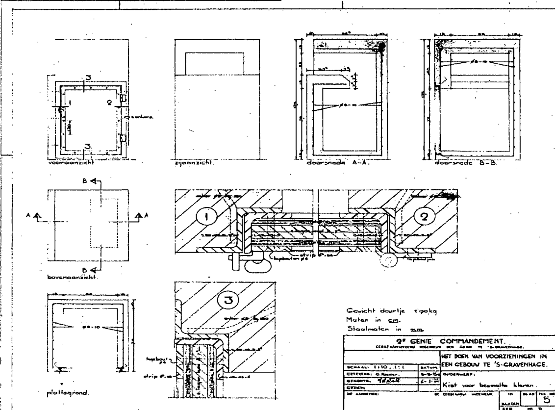
100. Ontwerptekening voor de kist voor besmette kleren, d.d. maart 1964. (Herkomst: Coll. digitale bestanden RVB)
