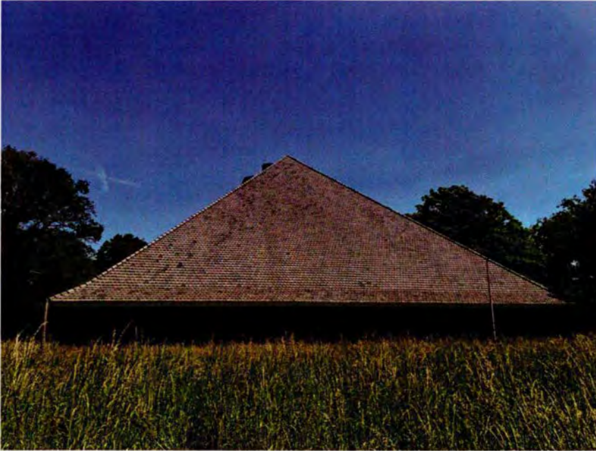
11. De bunker gezien vanuit het westen. Het dak rust aan deze zijde deels op zes betonnen en met baksteen omklede kolommen. Bij de aanpassingen van 1969 heeft men tussen de kolommen halfsteens dikke baksteenwanden gebouwd om de achterliggende ruimte beter te kunnen gebruiken.
