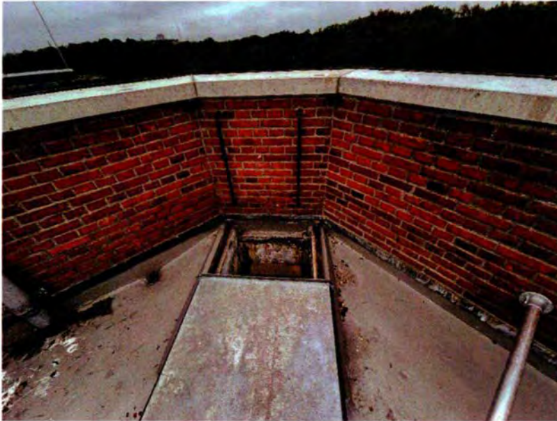
732. Het dakluik van de westelijke observatietoren. De constructie is identiek aan die van de oostelijke toren. Ook hier is een extra stalen reling geplaatst (2020) en de bodem vervangen tijdens de werkzaamheden van 2019.
